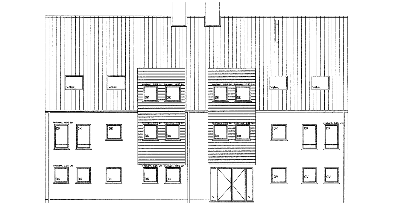
VOORGEVEL
