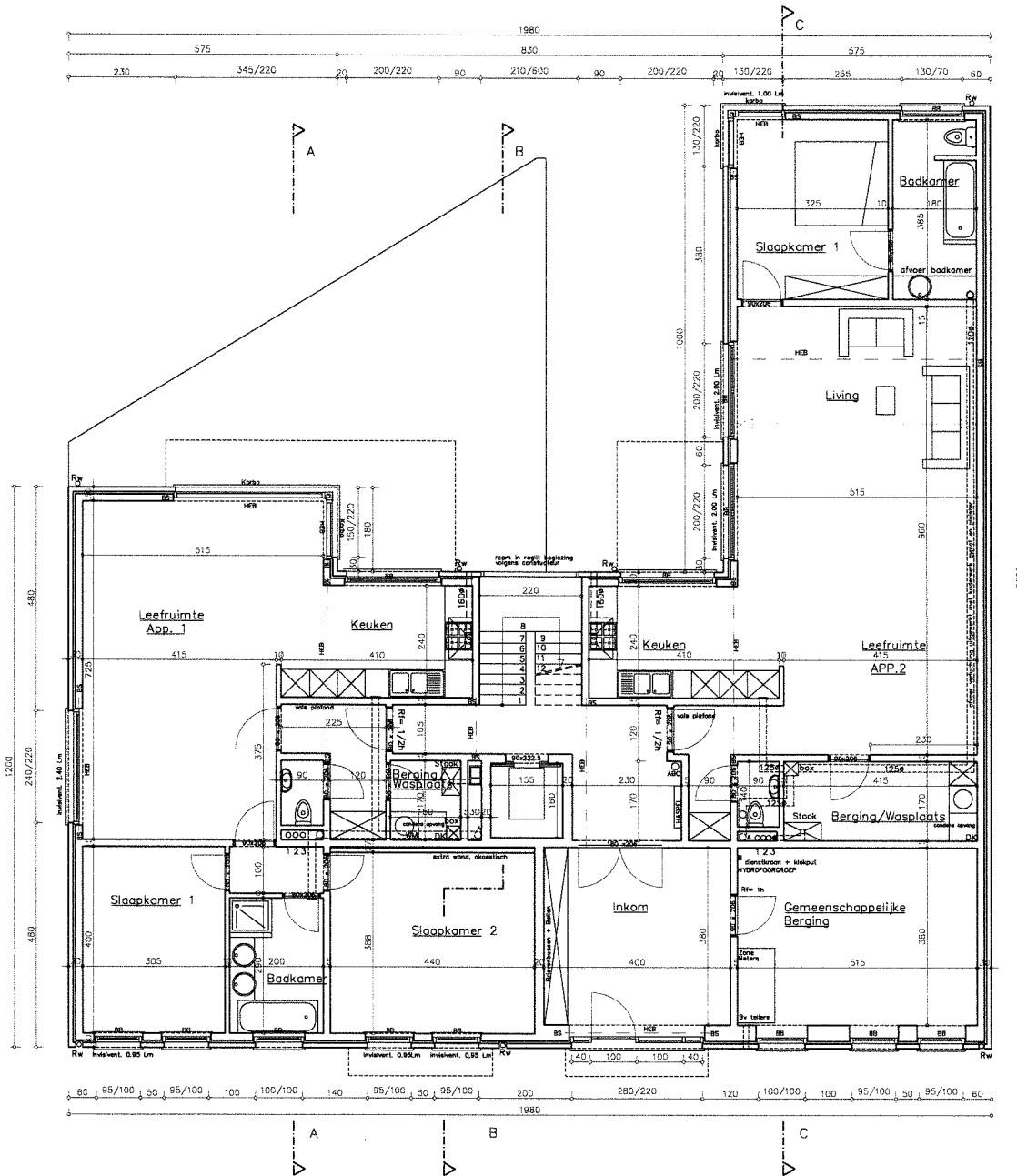
GRONDPLAN
