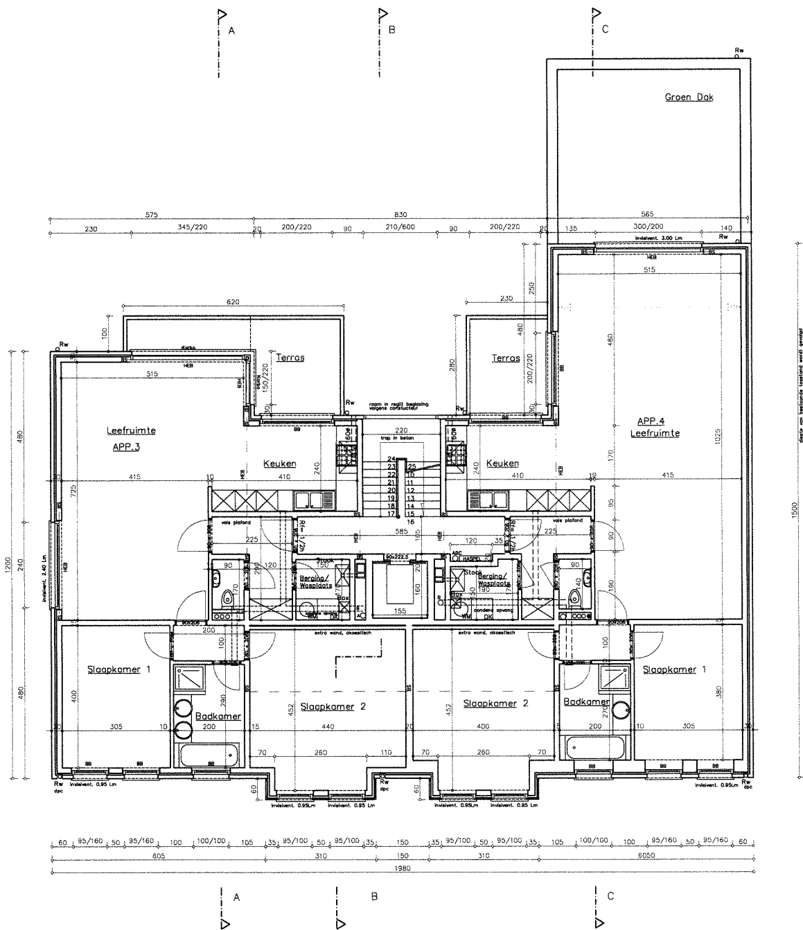
VERDIEPINGSPLAN
